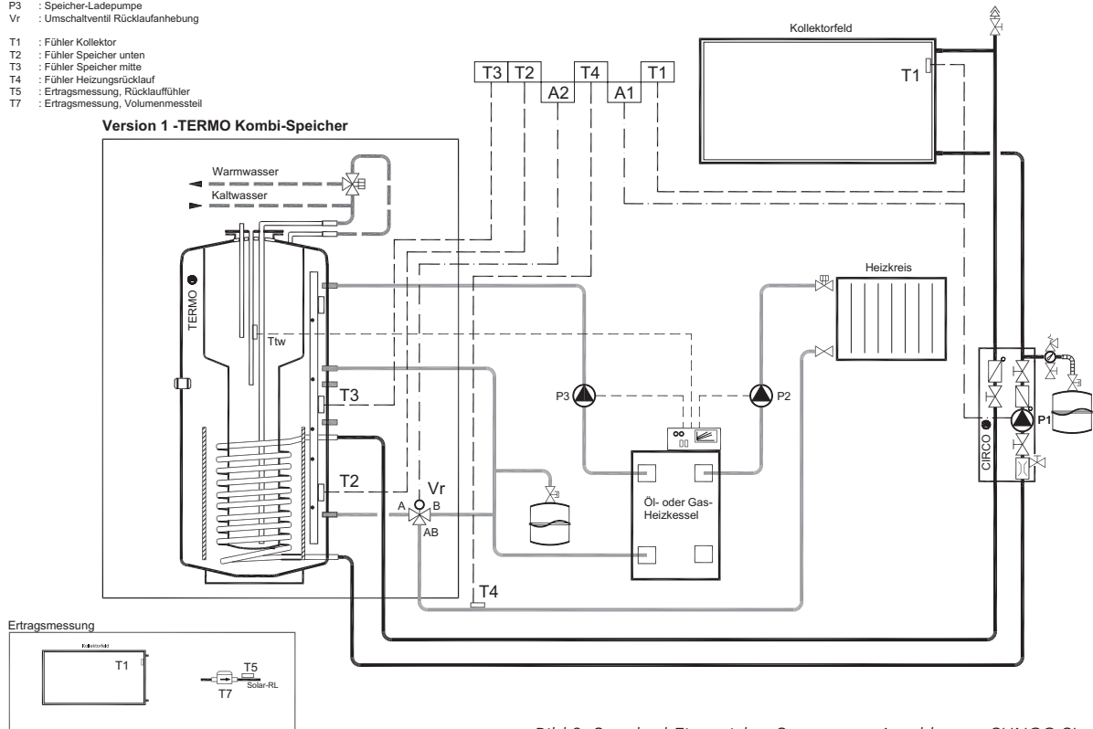
Bild 3 Standard-Einspeicher-System zum Anschluss an SUNGO SL
