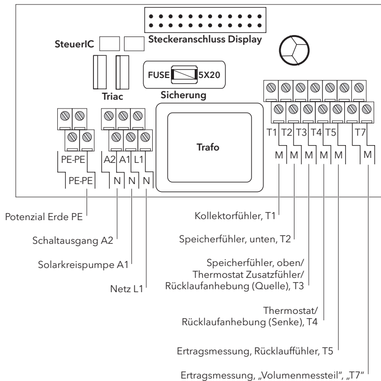
Bild 2 Reglerplatine SUNGO SL mit Klemmenbelegung für elektrischen Anschluss
