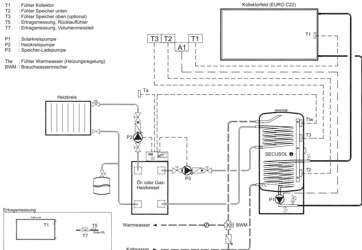
Bild 5 SECUSOL-System zum Anschluss an SUNGO SL
