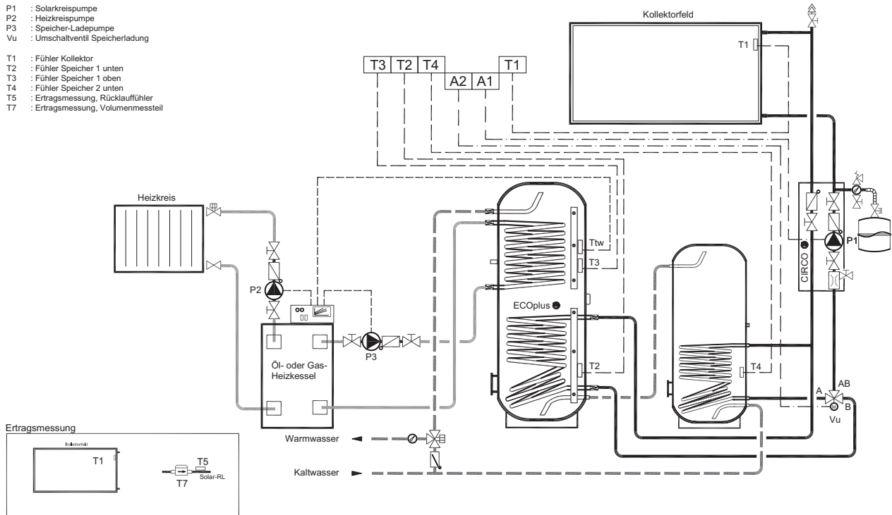
Bild 4 Standard-Zweipeicher-System zum Anschluss an SUNGO SL
