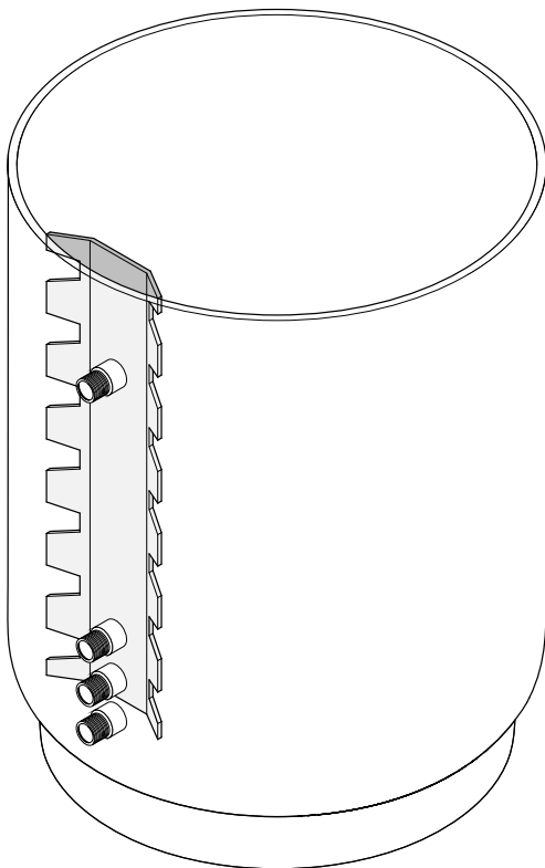
Abb. 8 Unterer Speicherbereich (geschnitten) mit innenliegendem Strömungsleitblech.
